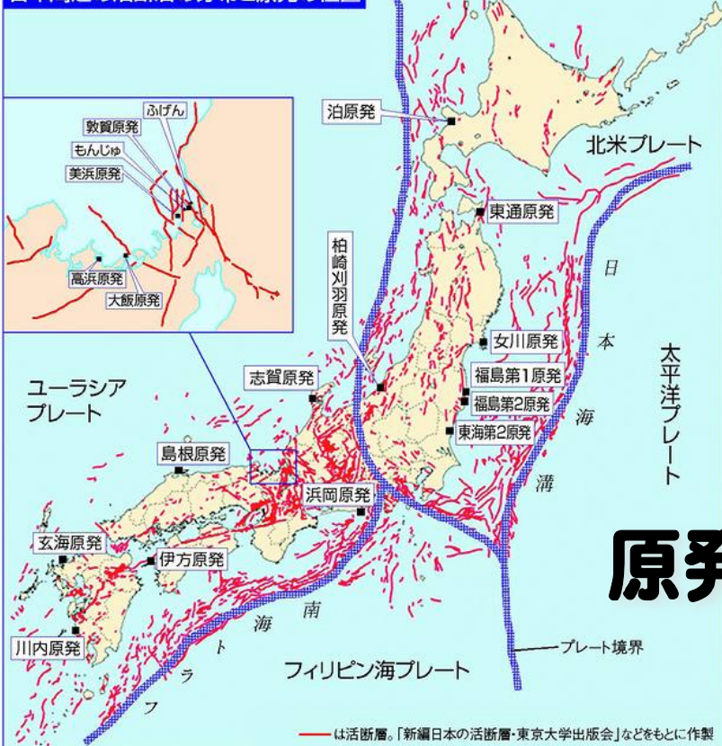
日本周辺の活断層の分布と原発の位置
